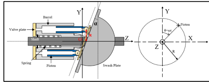
Figure 7 Schéma de principe d'une pompe à piston axiaux pour décrire la cinématique du piston
