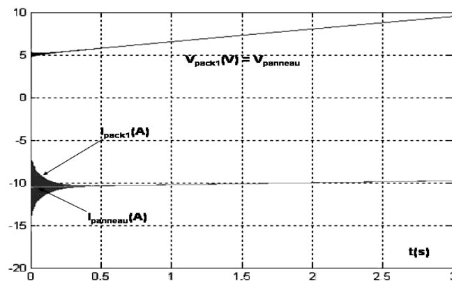
Fig. 9: Allures des tensions et courants du pack1 et du panneau solaire lors de la charge lente
